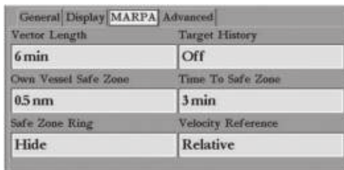
Меню настройки MARPA
